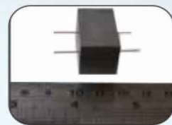
線切割超始孔加工 材質:模具鋼 L=18mm Φ=0.2mm
